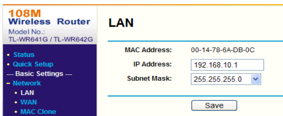
Figura A.2.2 Defina os parâmetros LAN
