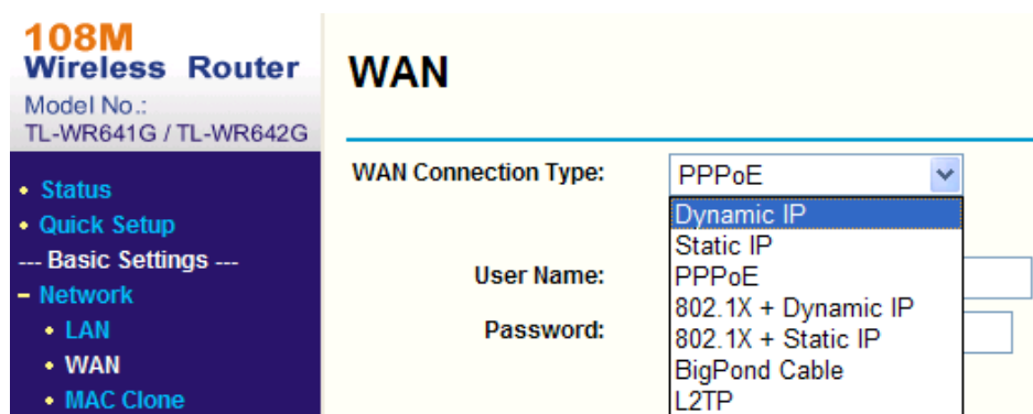
Figura A.2.1 Seleccione o tipo de ligação WAN
