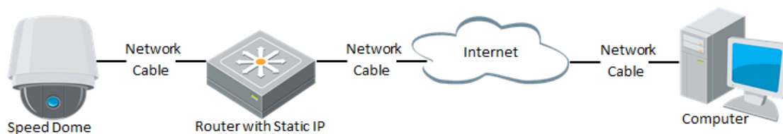
Figura 2-5 Acceso al domo Speed a través de un enrutador con IP estática
