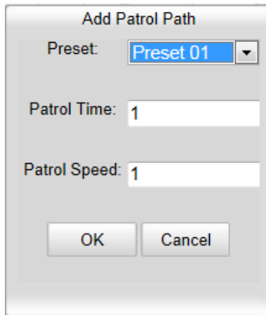
Figura 4-23 Añadir preajustes
