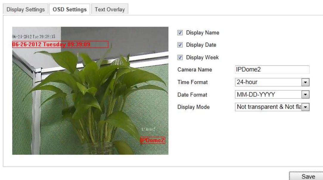
Figura 6-62 Ajustes OSD
