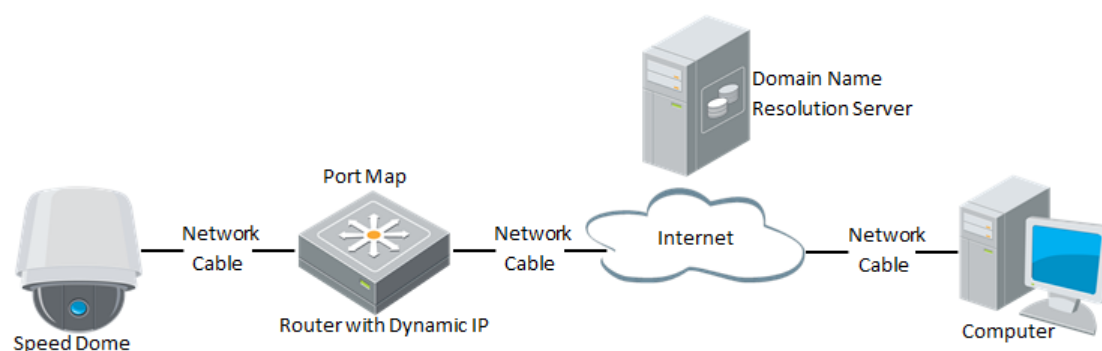
Figura 2-8 Resolución de nombre de dominio normal
