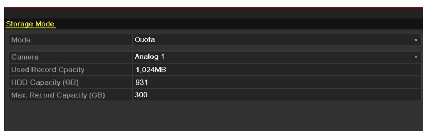
Figure 10.16 Configurer le quota d'enregistrement
