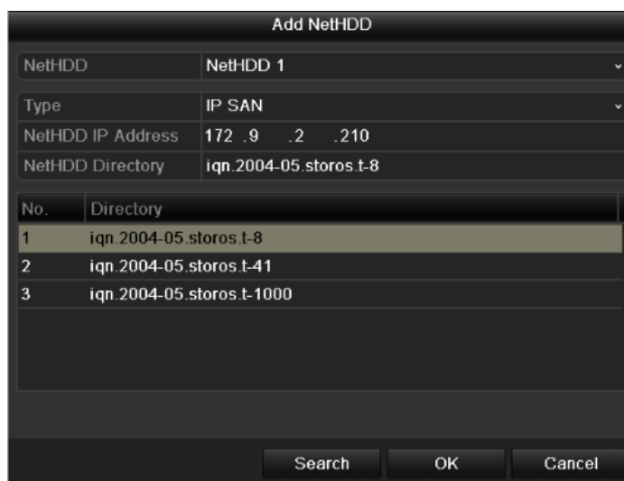
Figure 10.8 Ajouter un SAN IP
