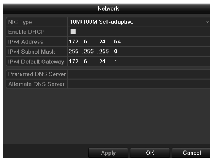
Figure 9.32 Paramétrage du réseau
