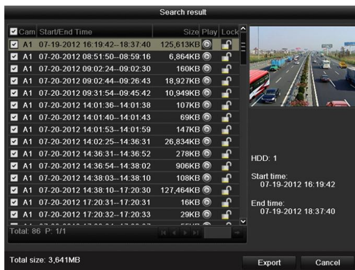
Figure 7.24 Résultat de recherche de vidéo normale pour sauvegarde
