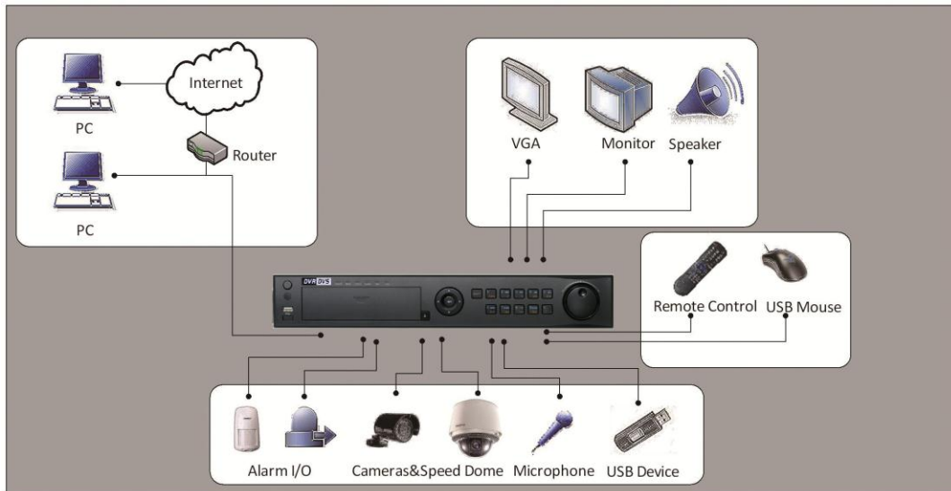
Fig 2 : Schéma du Raccordement du DVR
