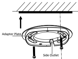
Fixer la plaque support d'entraînement du dôme
