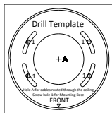
Gabarit de perçage
