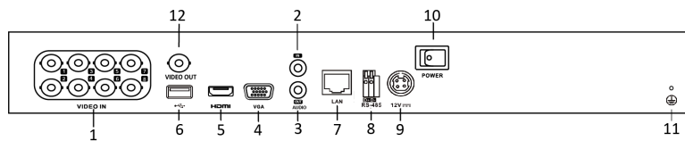
Figura 1–15 Panel posterior de la serie DS-7200HQHI-F2/N
