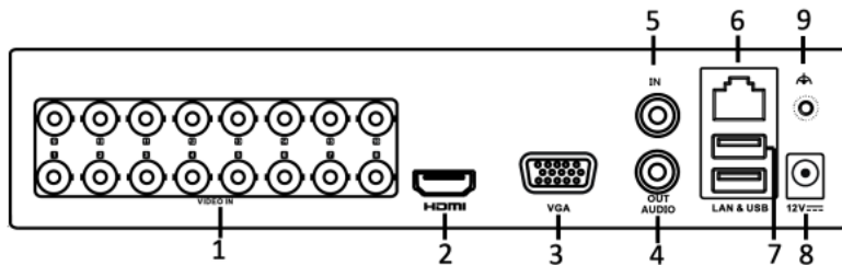
Figura 1–12 Panel posterior de la serie DS-7200HGHI-F (/N)
