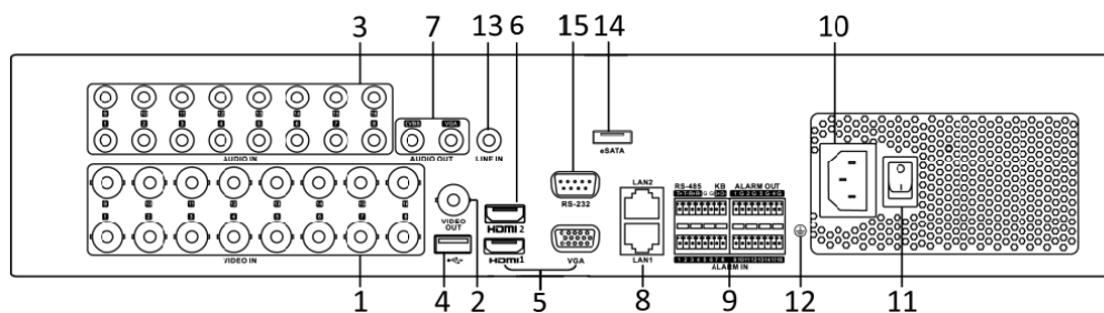
Figura 1–21 Panel posterior de la serie DS-9000HUHI-F8/N
