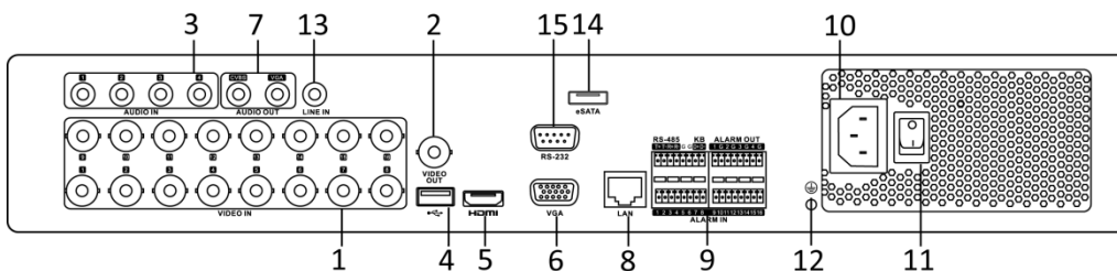
Figura 1–17 Panel posterior de la serie DS-7300HQHI-F4/N
