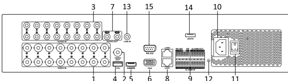
Figura 1–18 Panel posterior de la serie DS-8100HQHI-F8/N
