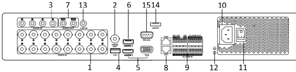
Figura 1–19 Panel posterior de la serie DS-7300HUHI-F4/N
