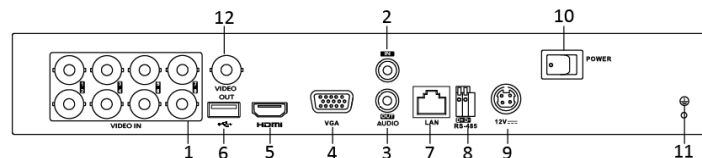
Figura 1–14 Panel posterior de la serie DS-7200HQHI-F1/N
