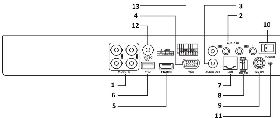
Figura 1–16 Panel posterior de las series DS-7200HUHI-F/N y 7600HUHI-F/N
