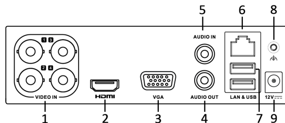
Figura 1-11 Panel posterior de la serie DS-7100
