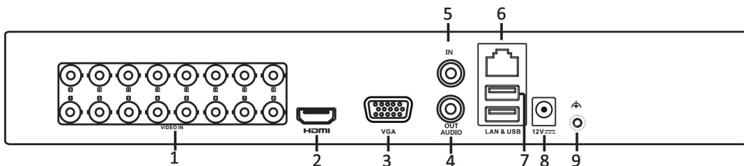
Figura 1–13 Panel posterior de la serie DS-7200HGHI-E
