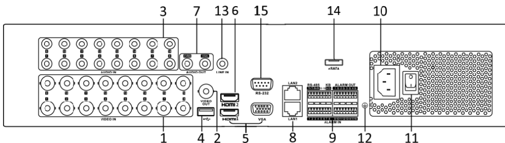
Figura 1–20 Panel posterior de la serie DS-8100HUHI-F8/N
