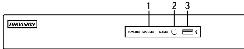
Figura 1-3 Panel frontal de la serie DS-7200HQHI-F/N
