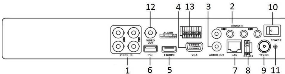
Figura 1-9 Pannello posteriore dell'unità DS-7200HUHI-K/P
