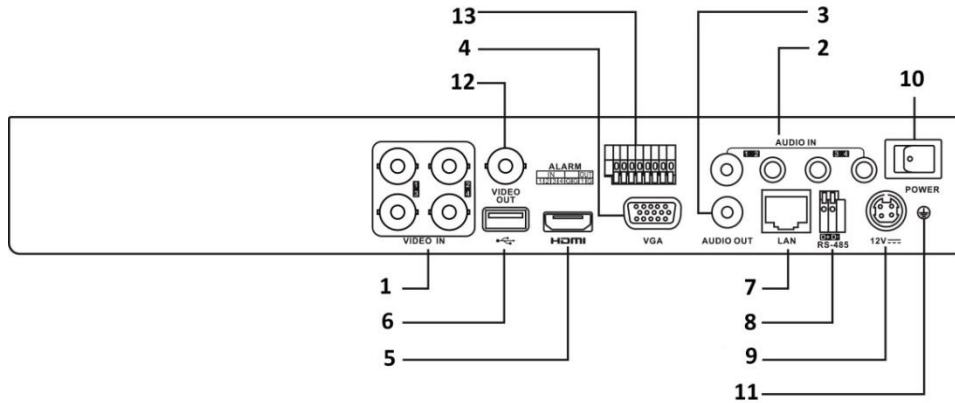
Figura 1–10 Pannello posteriore dell'unità DS-7200HTHI-K1
