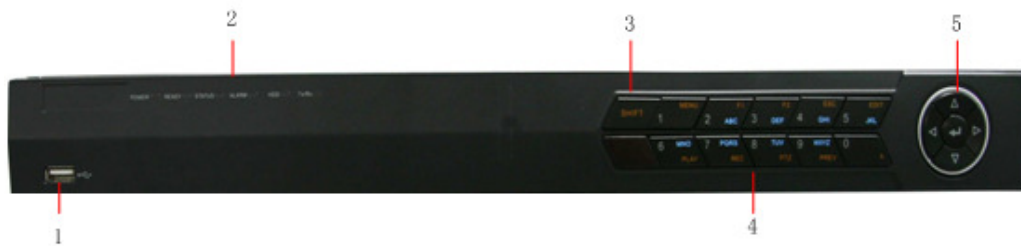
Figura3-2. Pannello frontale del DS-7608NI-S
