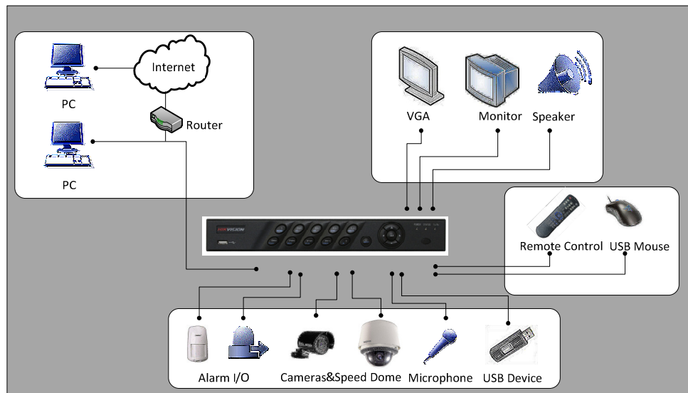
Fig 2: Layout dell’NVR/HVR e delle periferiche
