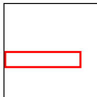
Afb. 7-2 Schijf initialiseren
