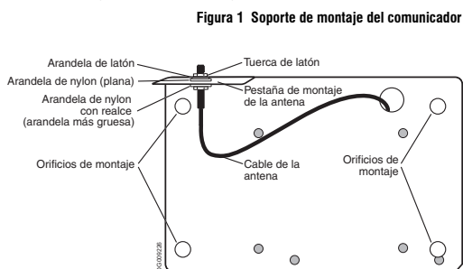
Figura 1 Soporte de montaje del comunicador
