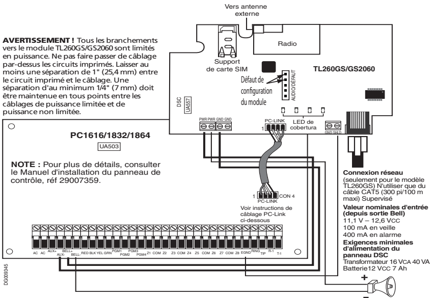
Figure 3 Schéma de câblage GS2060/TL260GS
