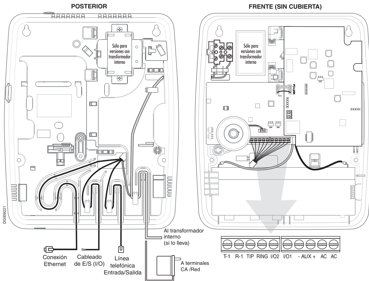
Figure 2-3 Detalles de montaje y cableado
