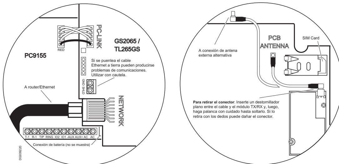
Figure 2-2 Detalles del cableado del módulo GPRS/Ethernet
