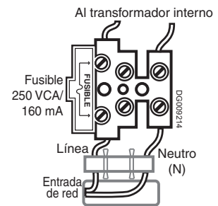
Figure 2-1 Bloque de fusibles de red
