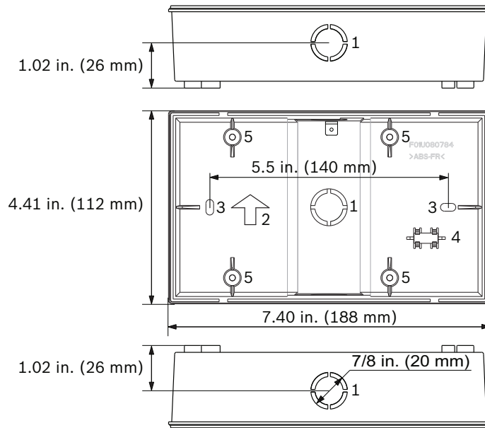
รูป 4.2 กล่องรองรับด้านหลังของตัวแจ้งเตือนระยะไกล FMR-1000-RA
